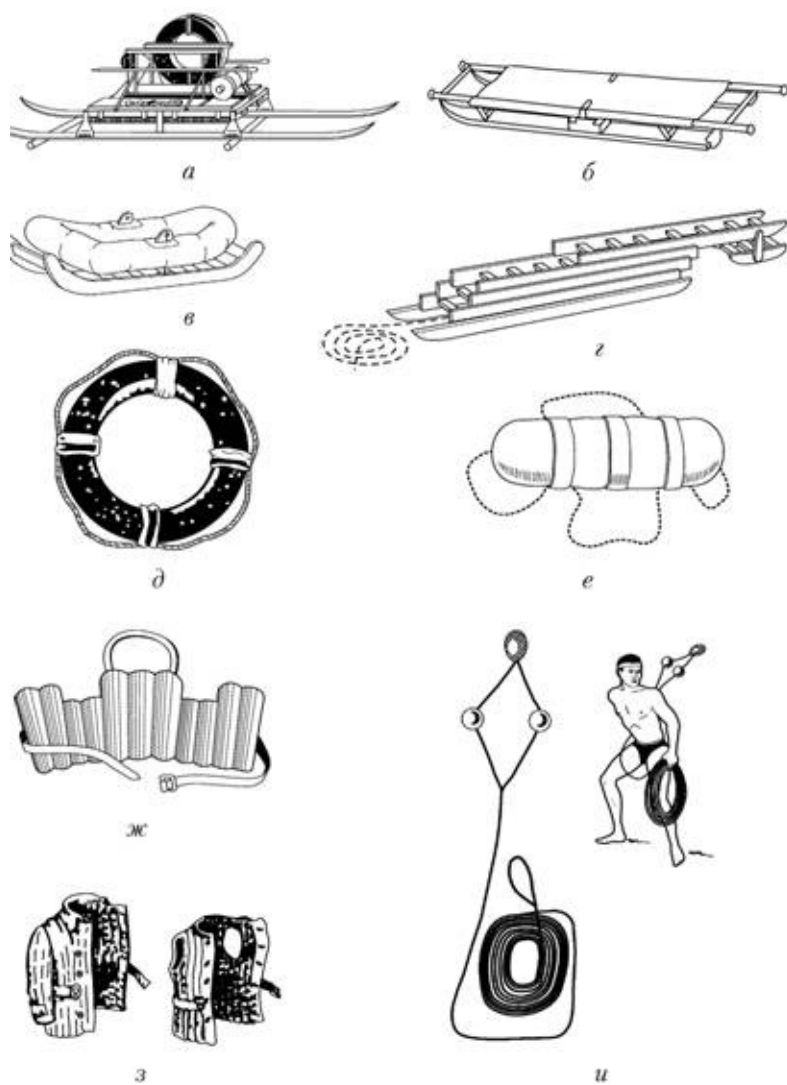
Рис. 82. Табельные спасательные средства:
